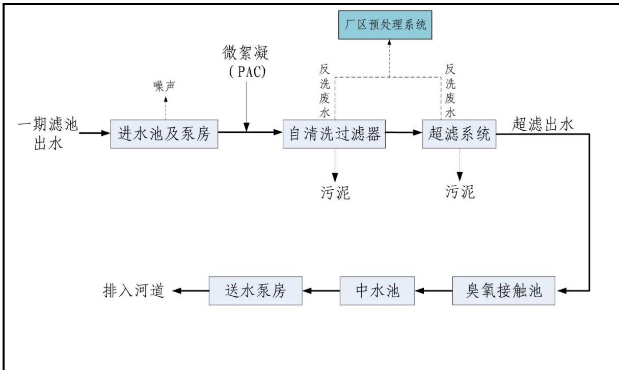
图 2-4 中水系统提标改造工程二期工程工艺流程图 (38000t/d)
